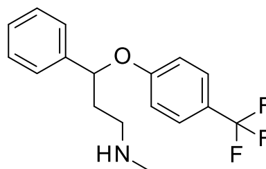
Figura 8 Estrutura molecular da fluoxetina
