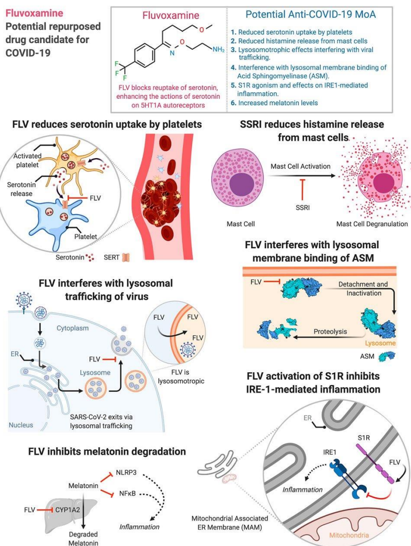
Figura 7 Mecanismos potenciais de benefício do uso de fluvoxamina em pacientes com quadro de COVID-19 112
