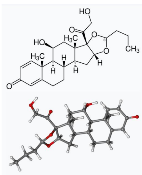
Figura 9 Budesonida – estrutura molecular
